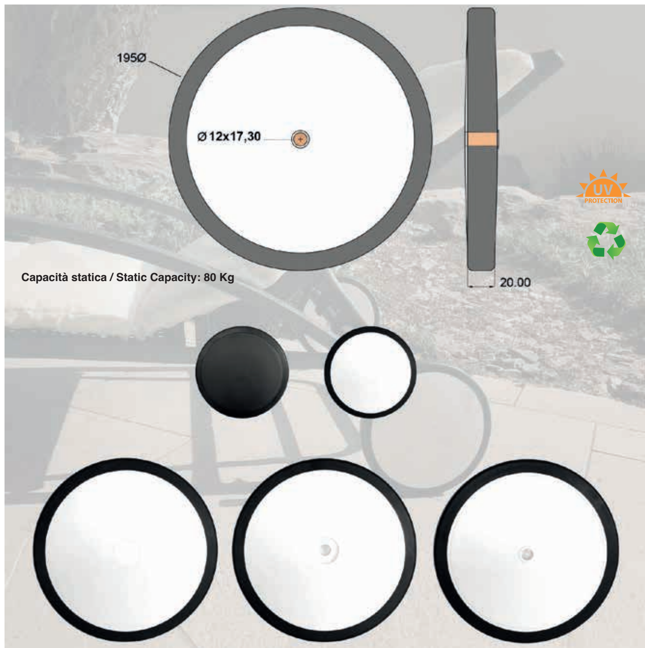
Fronte con e senza tappo centrale Front with and without central cap
